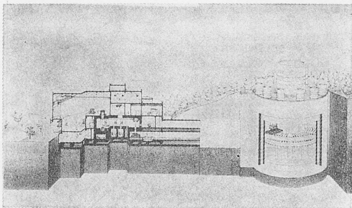
図7 高レベルガラス固化体貯蔵施設の概念図（平成元年版「原子力白書」より）
