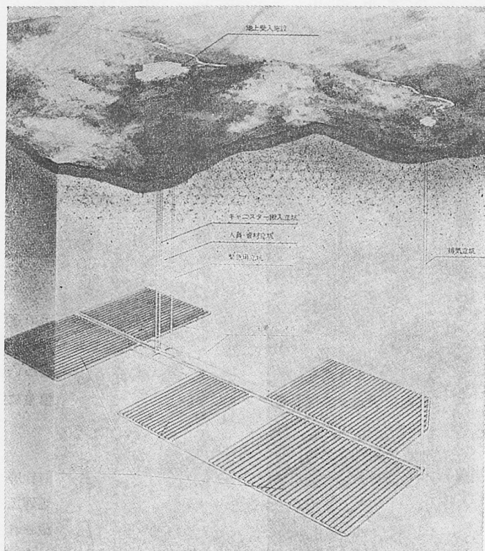
図9 高レベル廃棄物地層処分場の概念図（平成元年版「原子力白書」より）
